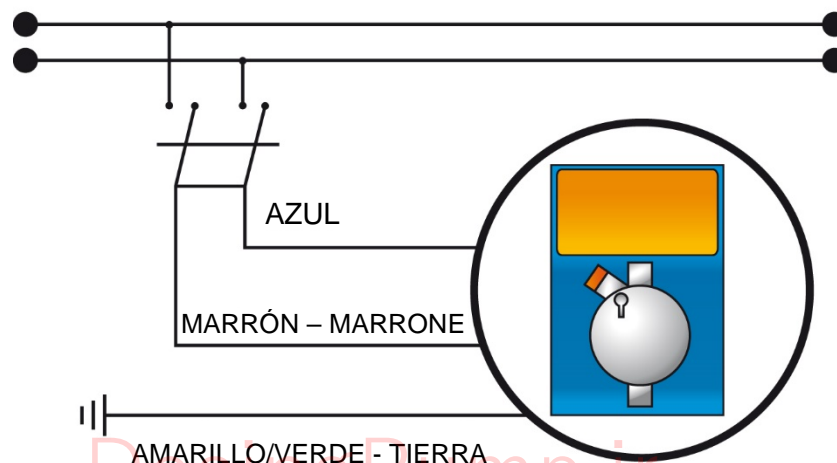
Fig. 3 - Conexión eléctrica
