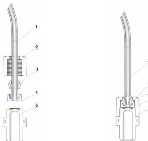
Abb. 4 - Anschluss der Flüssigkeitsleitungen
